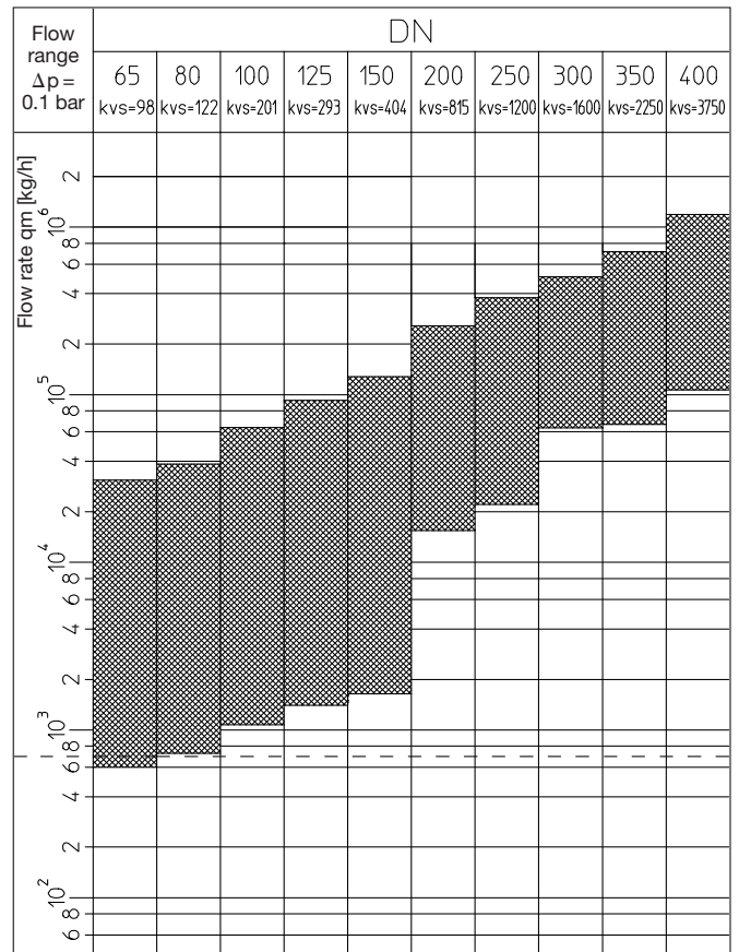
“Hydrocontrol VFC/VFR/VFN/VGC”
